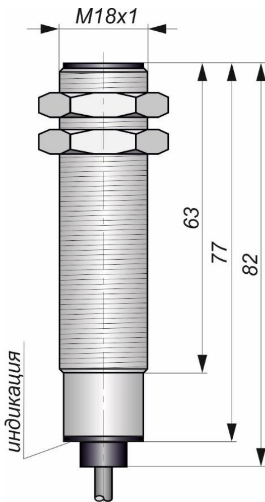
Габаритный чертеж
